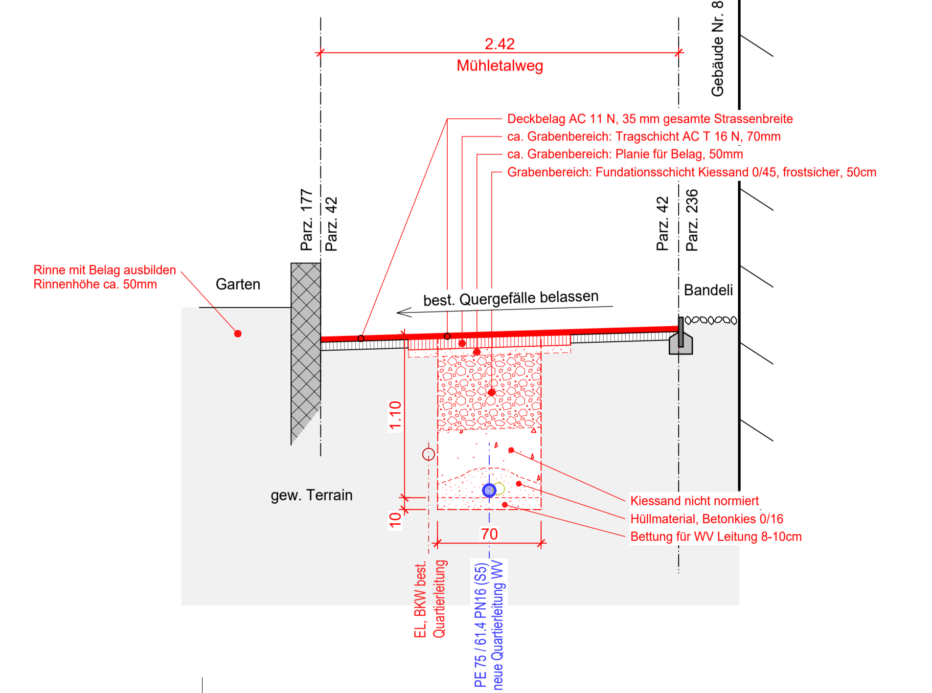
Querprofil C-C, 1:25
