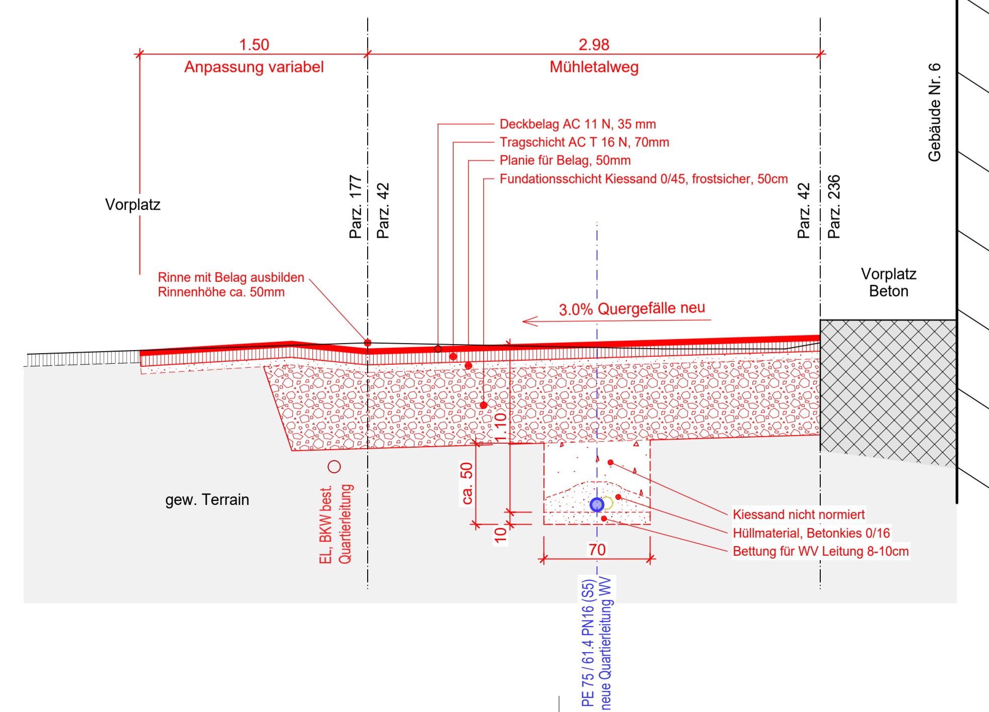
Querprofil B-B, 1:25
