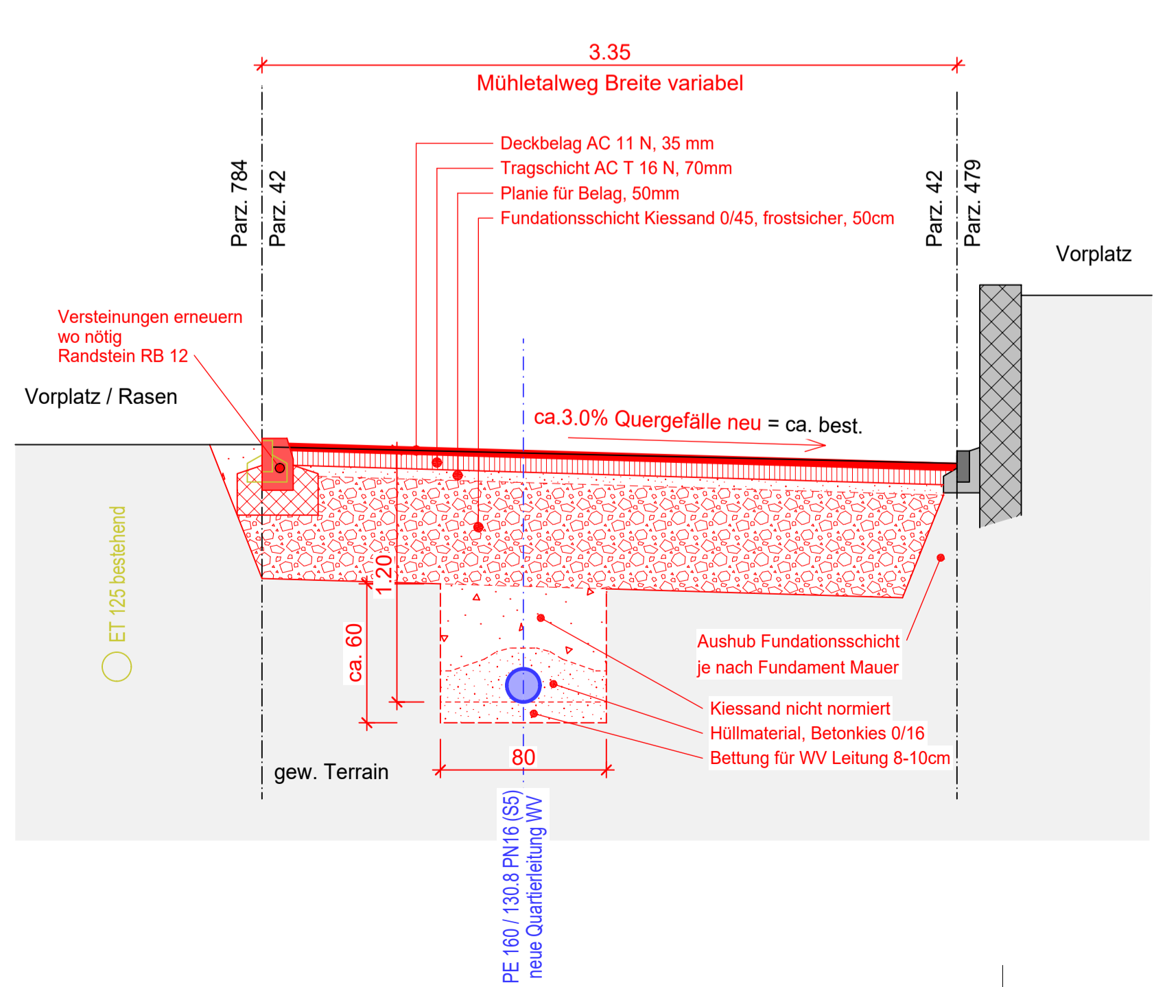
Querprofil A-A, 1:25
